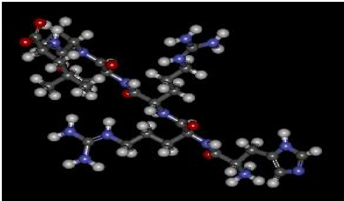
Fig. 3-MHC Molecule
